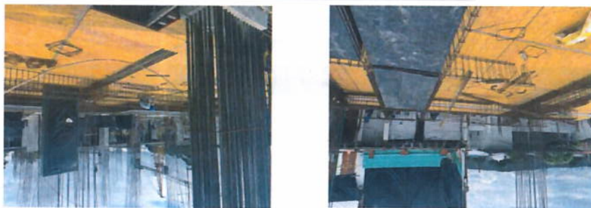
ARMADO DE ACERO DE REFUERZO PARA VIGAS DE ENTRE PISO ENTRE EJES AF Y EJES 7 AL 9
